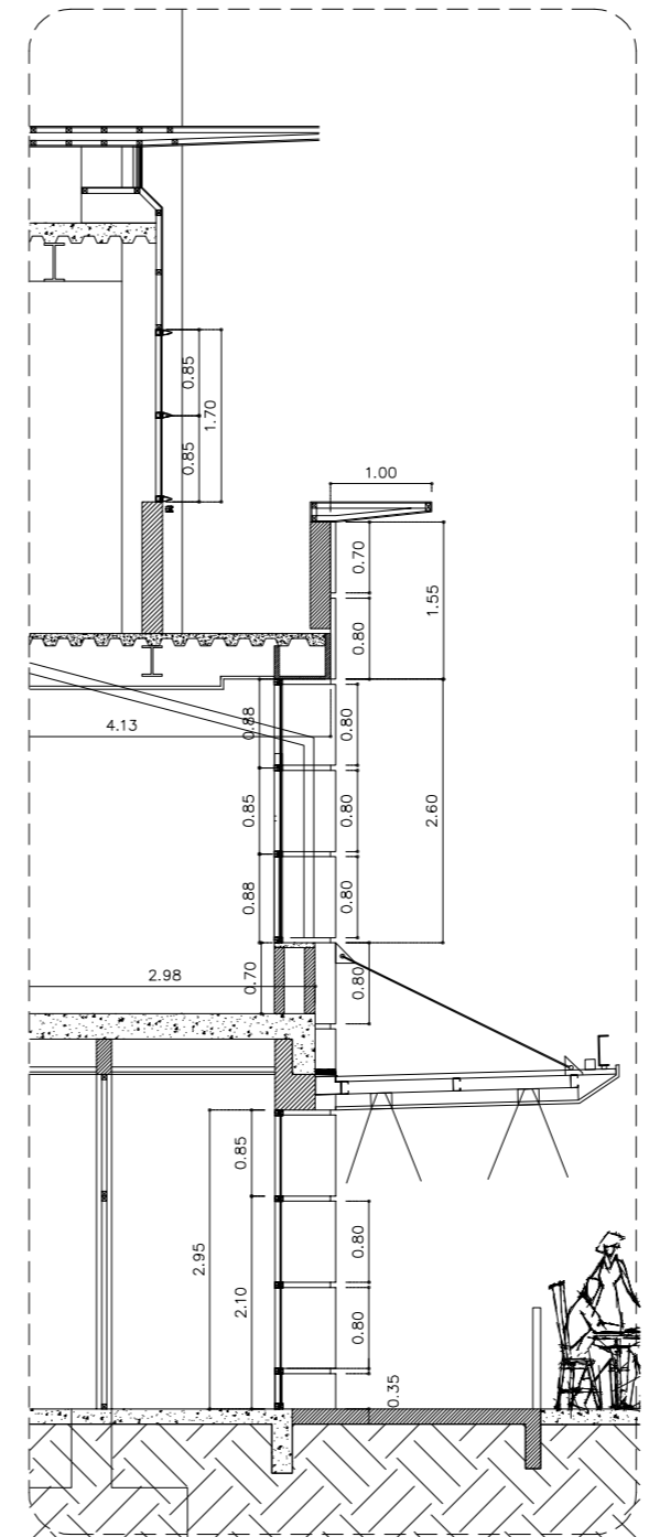
CORTE A-A'
