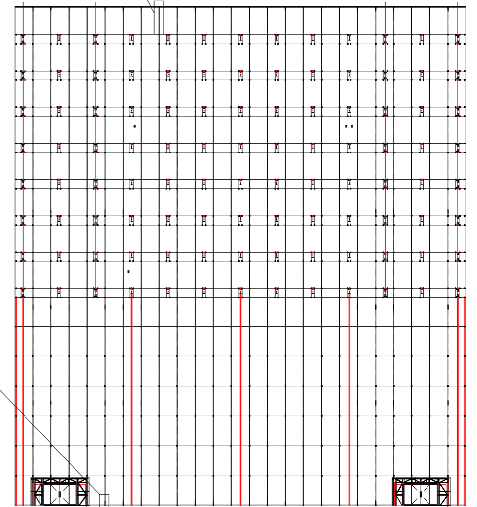
FACHADA ESTE
